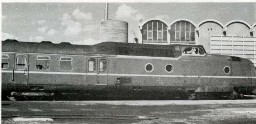
Lyntog litra Ma nr 461 Diesel-hydraulisk kraftoverføring Max hastighed 160 km/t 1 x 1100 HK + 1 x 296 HK Længde 19,20 m Tjenesteklar vægt 51 tons Elvarme Byggeår 1963
