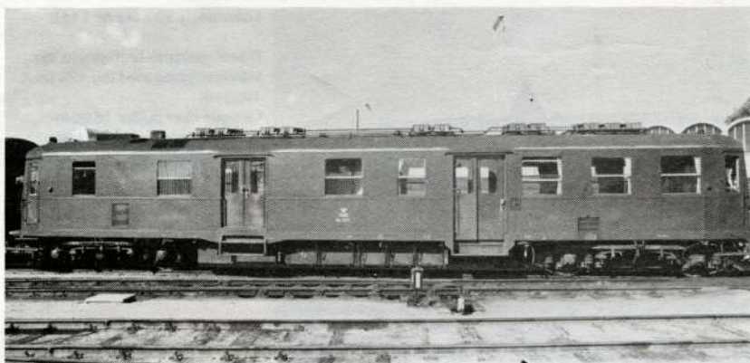
Motorvogn litra Mo nr 1883 Diesel-elektrisk kraftoverføring Max hastighed med tog 120 km/t 2 motorer a 250 HK 37 siddepladser Længde over puffer 20,90 m Tjenesteklar vægt 65,1 tons Dampvarme Byggeår 1957
