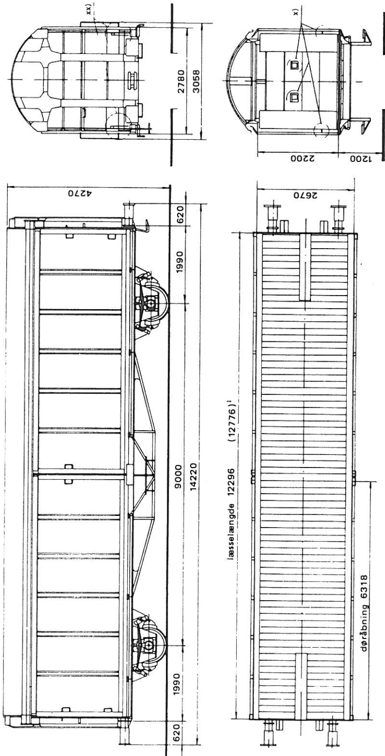
Hbikks-tt 237 2 000 - skala 1:100
